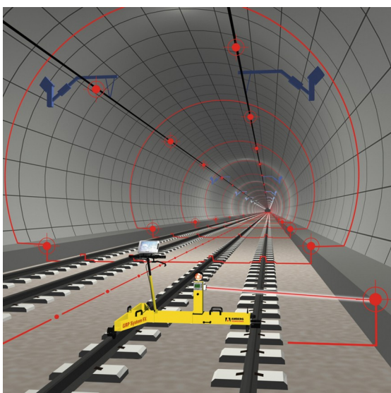
图 1: 间隙测量
