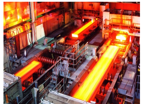
Abb 2: Stahlbrammen
