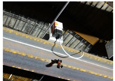
Abb 2: Dimetix Laser Sensor montiert an Querstrebe
